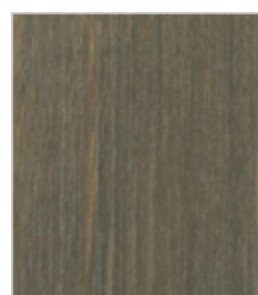
Горная лава 7184
