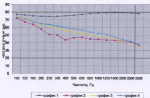
Уровни ударного шума под перекрытием
